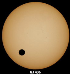
GJ 436
