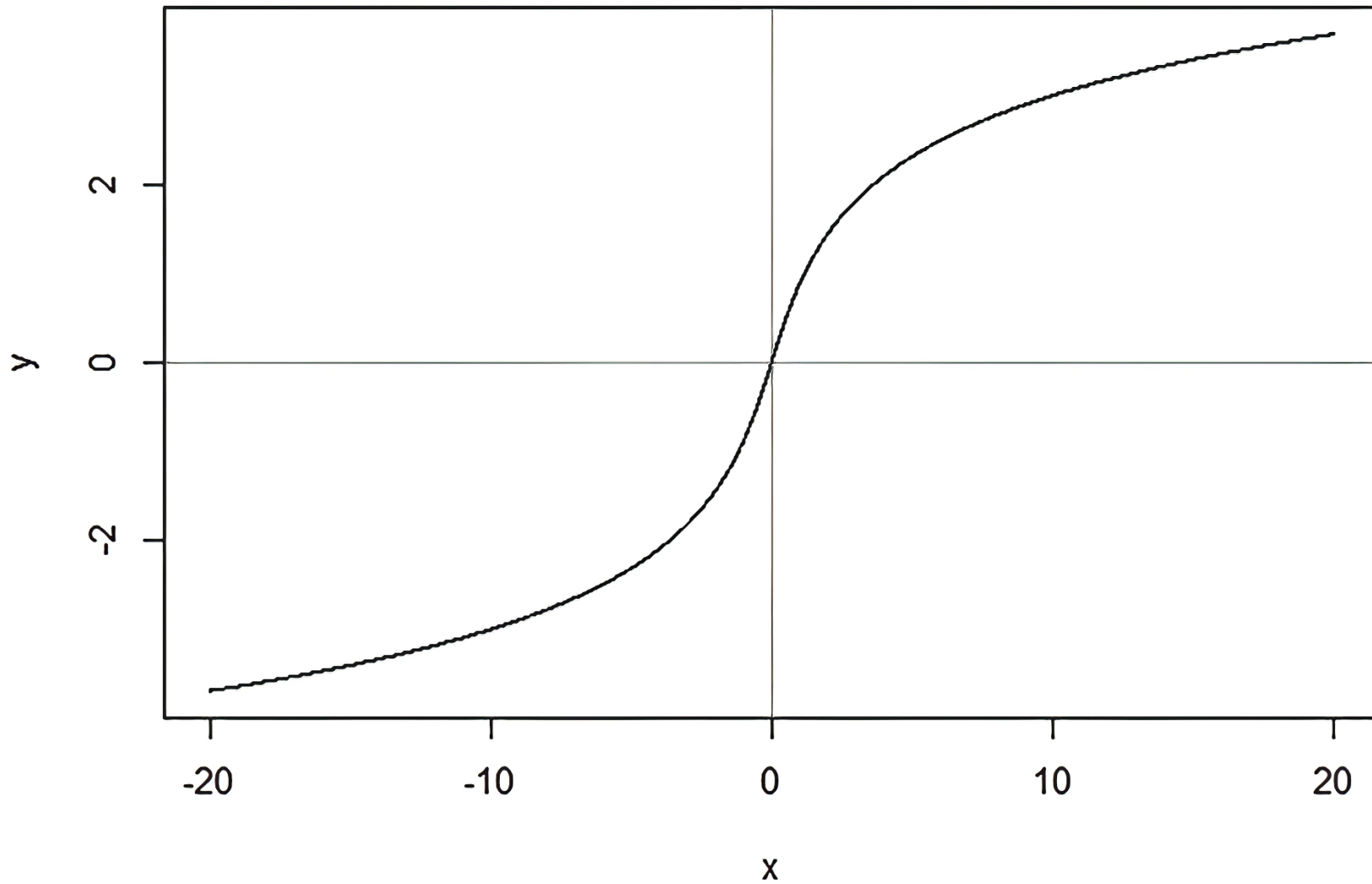
Arcsinh(x)
